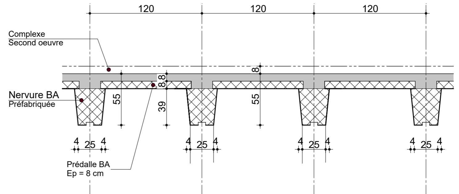
Coupe type sur plancher (Variante)
