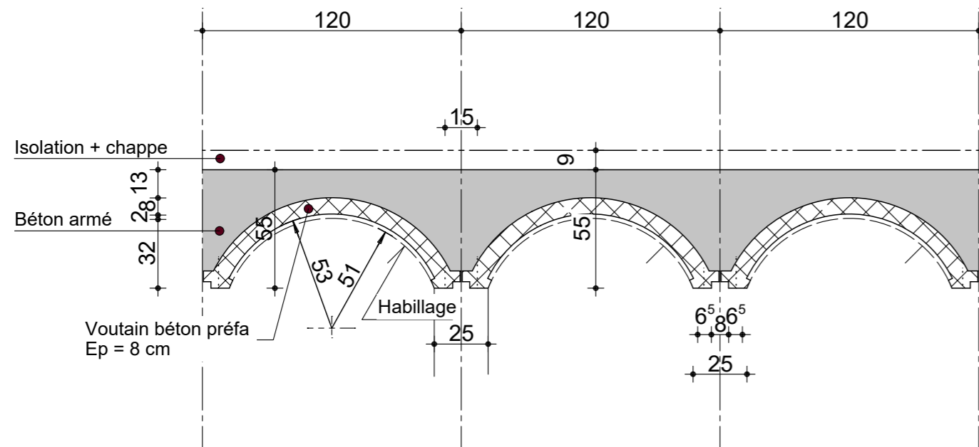
Coupe type sur plancher Voutains
