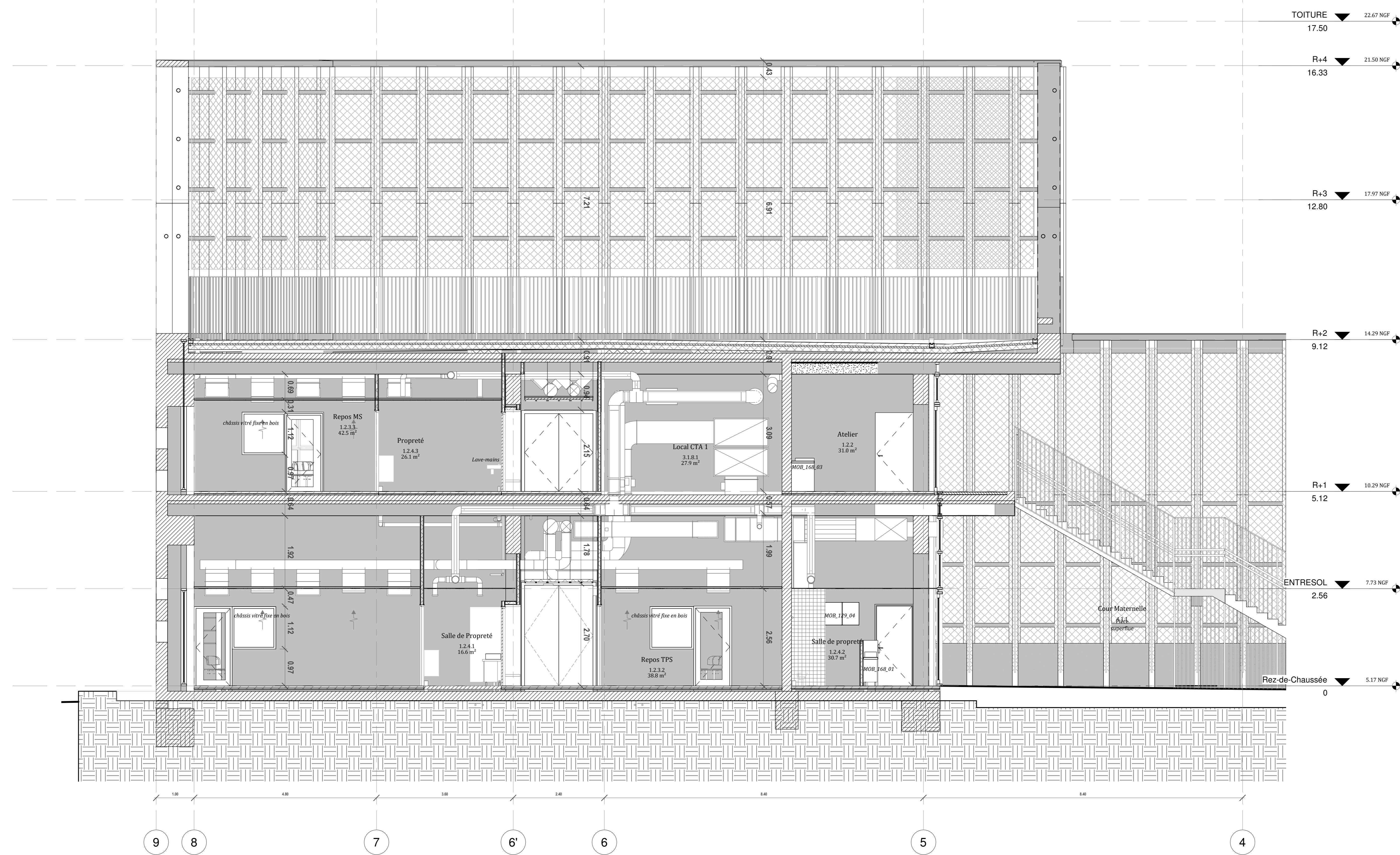
COUPE 16 1 : 50
