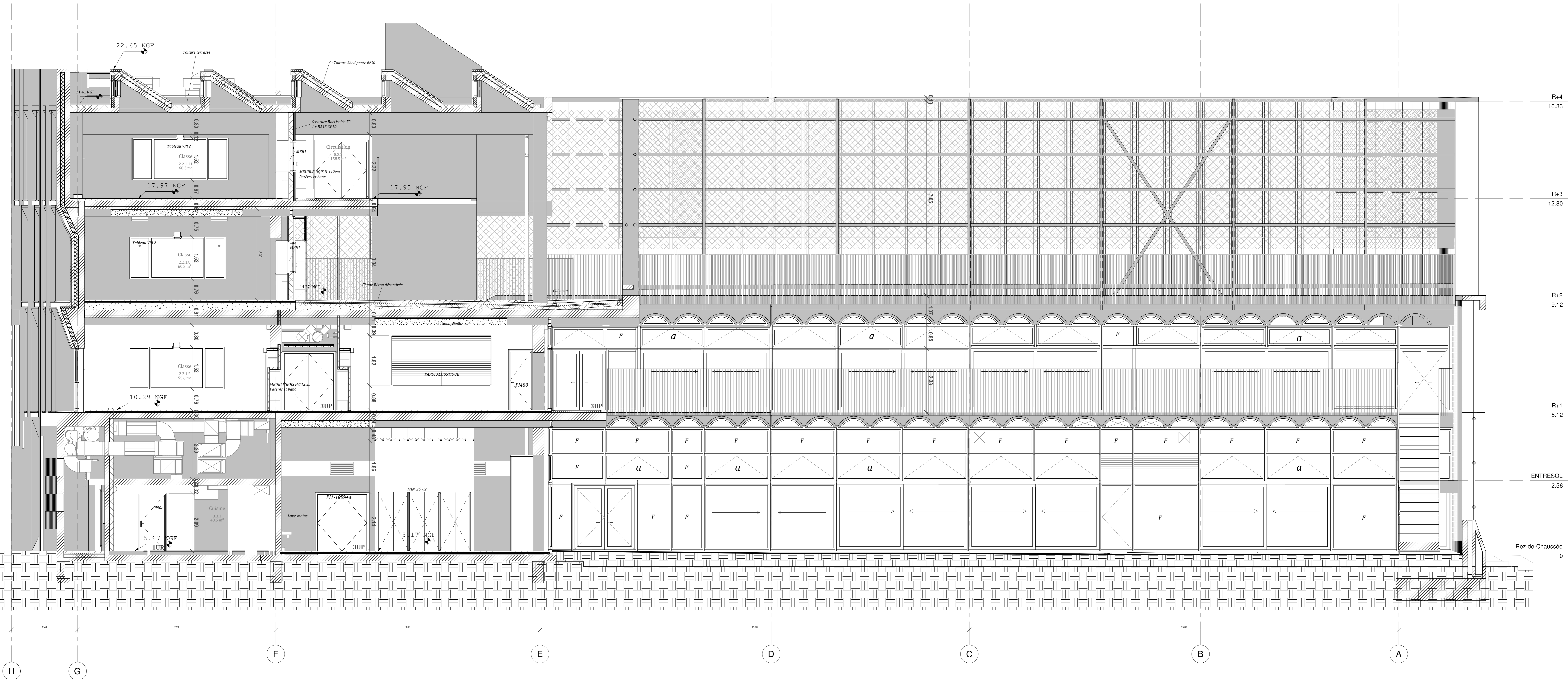
COUPE SUR ELEMENTAIRE ET COUR MATERNELLE 1 : 50
