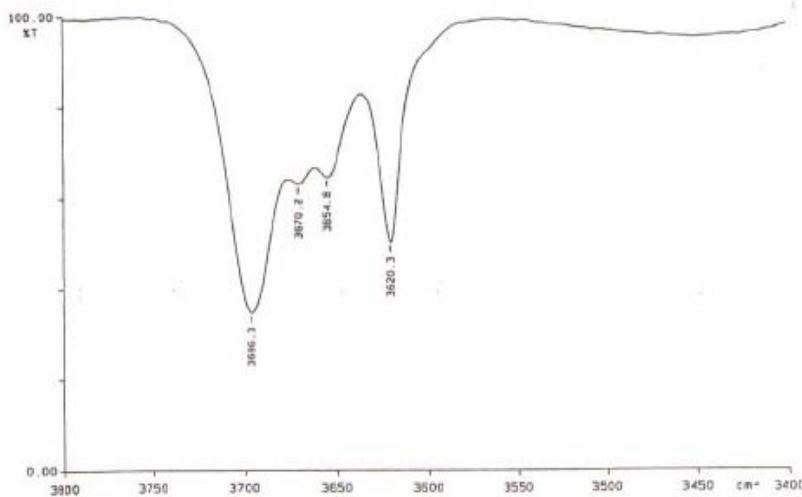
Spectre de la suspension au Nujol dans la région comprise entre 3800 et 3400 cm -1
